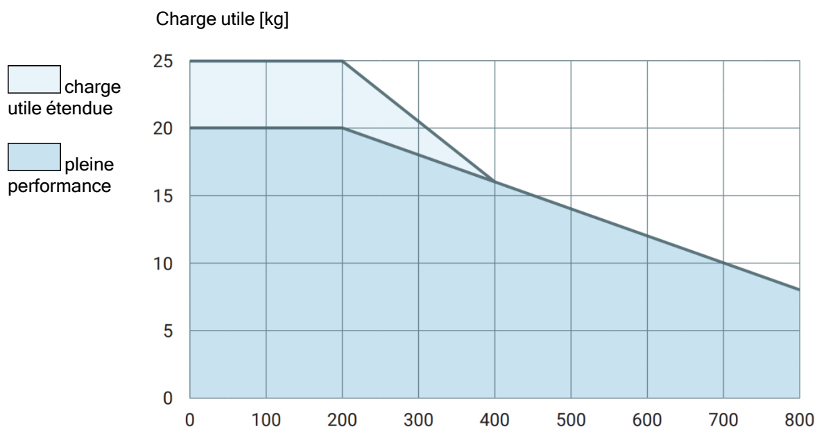
Décalage du centre de gravité [mm] La relation entre la charge utile nominale et le décalage du centre de gravité.
